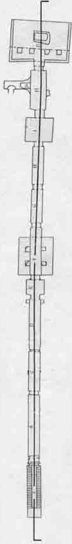
a) plan et coupe de la tombe k. v. 47 Siptah à la Vallée des Rois (D'après K. R. Weeks, Atlas of the valley of the kings, le Caire, 2000, sheet 61/72). Localisation en J1 de l'orifice de communication avec la k. v. 32 (Ja).
