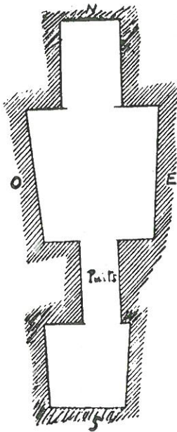
Figura 2.- Plano de las cámaras de la tumba n.º 2 de la necrópolis de Tehneh. (A.S.A.E. XXVI, 1926, 34, fig. 2)
